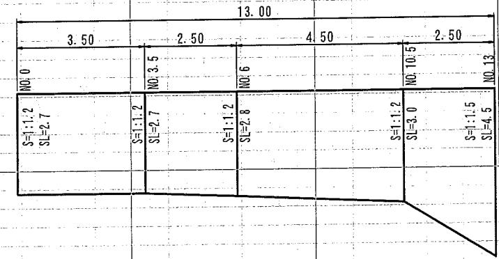
植生工展開図 S=1:100
