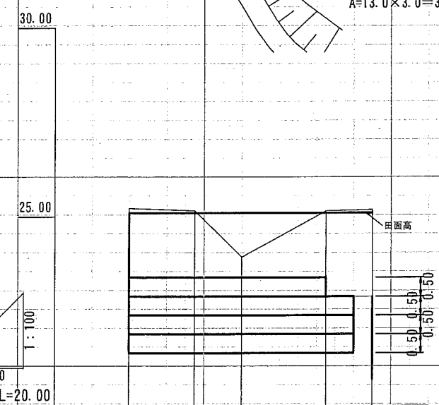
横断面図 S=1:100
