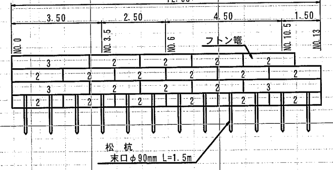
フトン管配置図 S=1:100
