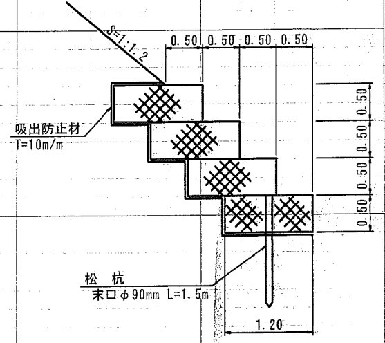
フトン管詳細図 S=1:50
