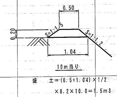
畦畔工 S=1:40
